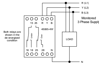
CONNECTION DIAGRAM DIAGRAMME DE CONNECTION SCHALTBILDANSCHLUSS
